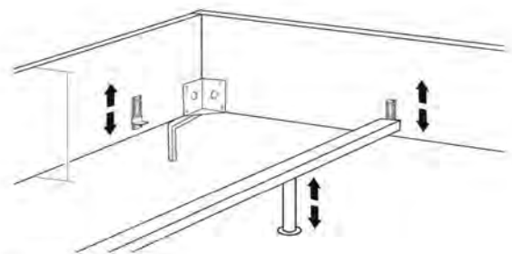
Einlegetiefen
